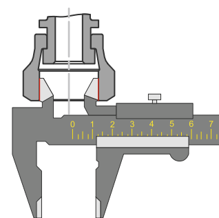
Измерение резьбы по наружному диаметру
